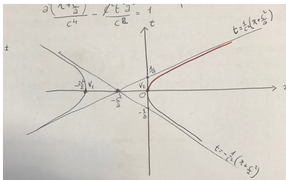
Figura 2: Diagramma orario del moto iperbolico.
