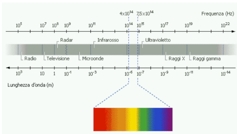
Figura 1: Spettro elettromagnetico.
